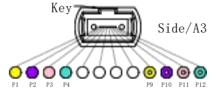
光缆参数 Cable Parameters
