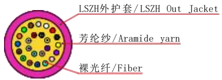
光缆示意图/Optical cable Diagram
