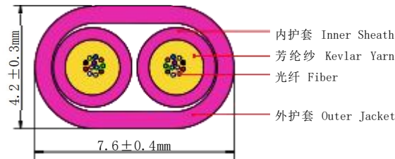
光缆示意图 Optical cable Diagram
