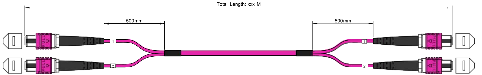
光缆示意图 Optical cable Diagram
