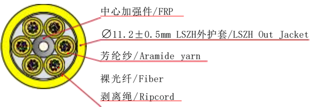
光缆示意图 Optical cable Diagram
