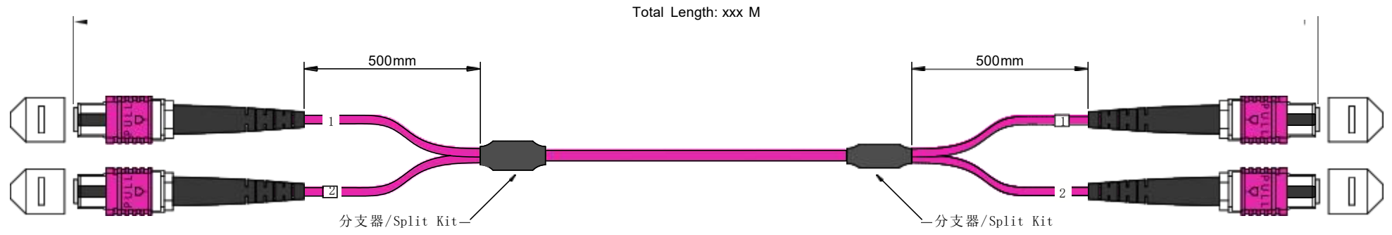
光缆示意图 Optical cable Diagram
